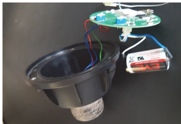
Rys. 4. Obudowa z płytą główną i czujnik
